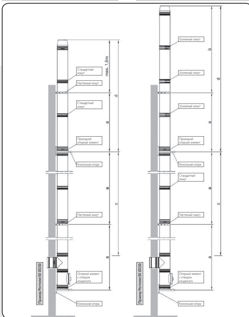
PERMETER50 Ø130-Ø250
