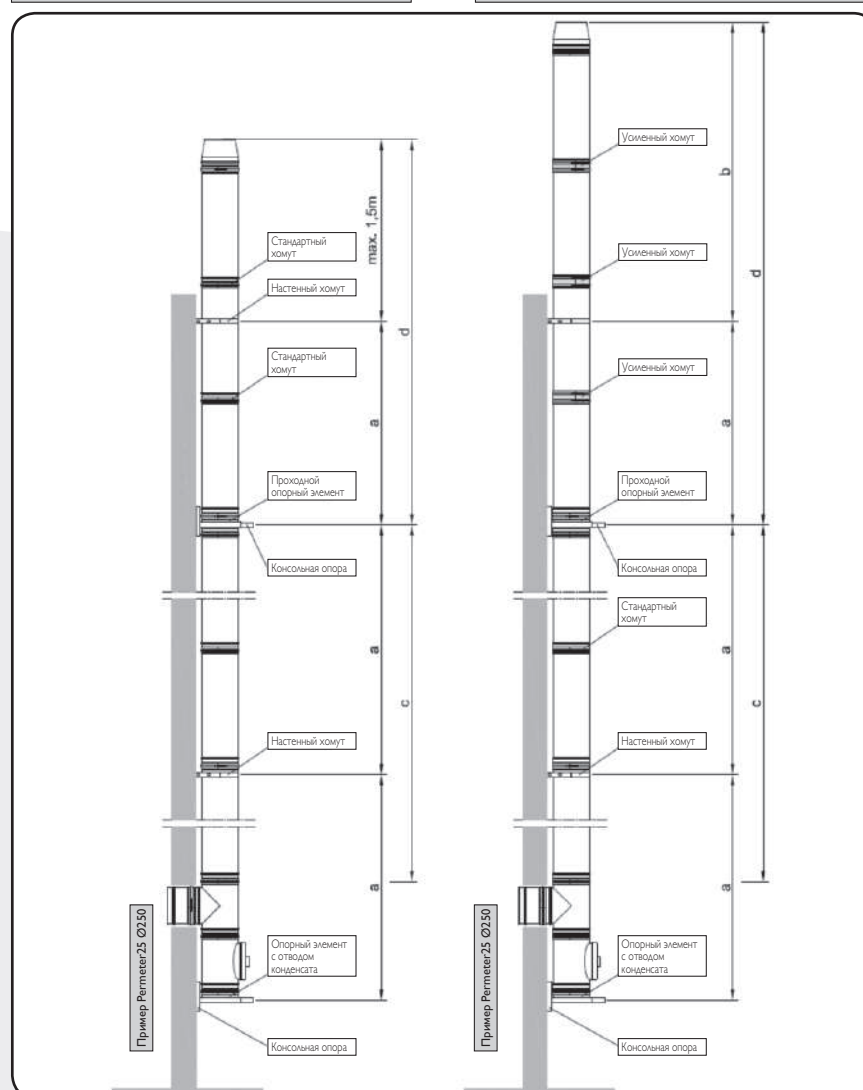
PERMETER25 Ø130-Ø250
