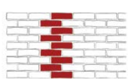
Ложковая в полкирпича
