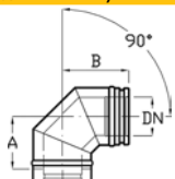
Отвод 90° + хомут
