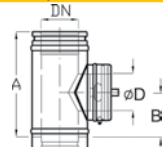
Тройник прочистки + хомут (T450 NI)
