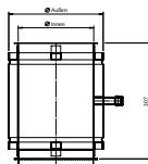
Элемент трубы с отверстиями для анализа газа
