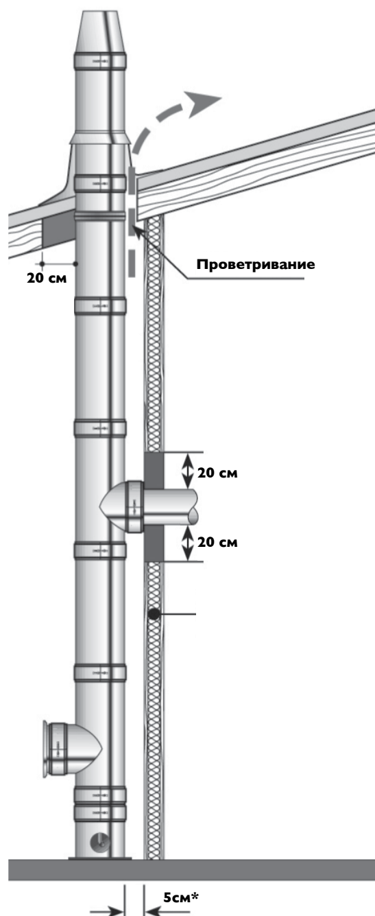
Отступы от горючих конструкций при проходе дымохода через стены и кровлю
